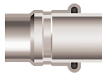
Przekrój połączenia po zaprasowaniu
