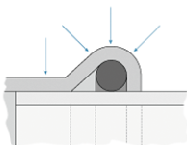
rys. Kierunki nacisku w połączeniu „press”
